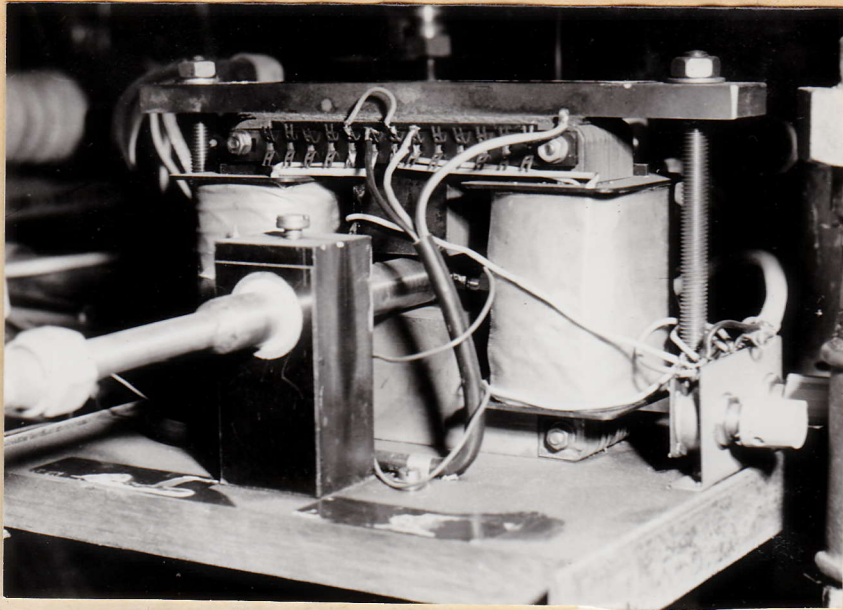
Bild 7 : Induktiver Durchflußmesser im eingebauten Zustand ( Zuströmrichtung )
